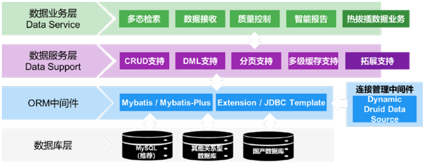
图 17 平台数据库方案
